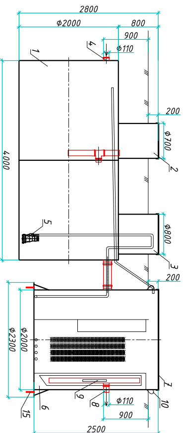
Разрез 1-1
